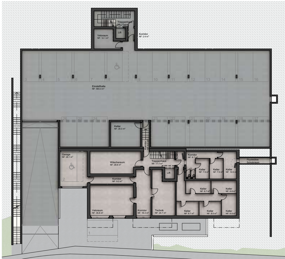
Keller Haus A und Einstellhalle 2. Untergeschoss
